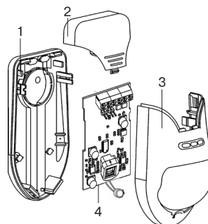
Рисунок 3 – Конструкция извещателя
