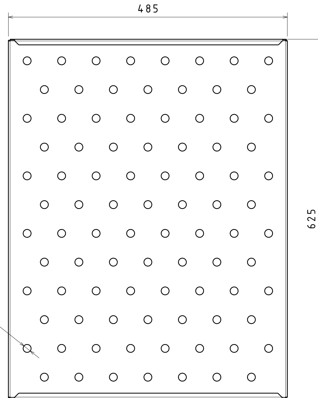
Вид снизу Масштаб: 1:4
