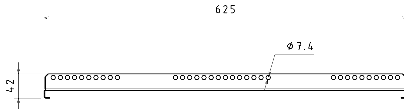
Вид справа Масштаб: 1:4
