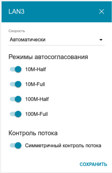
Рисунок 107. Окно изменения настроек порта маршрутизатора.
