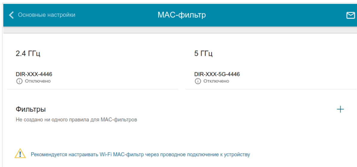
Рисунок 97. Страница для настройки MAC-фильтра для беспроводной сети.
