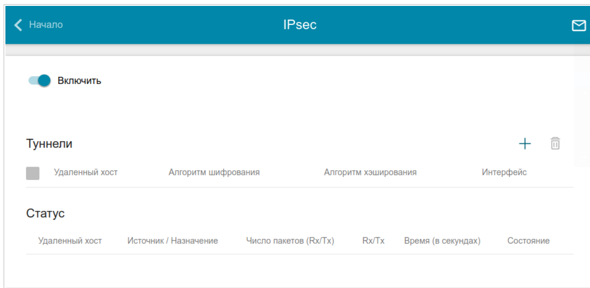
Рисунок 121. Страница Дополнительно / IPsec .
