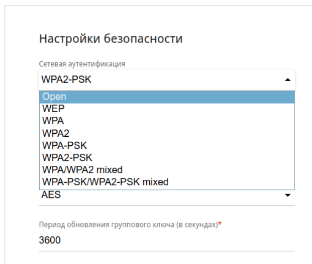
Рисунок 85. Типы аутентификации, поддерживаемые маршрутизатором.
