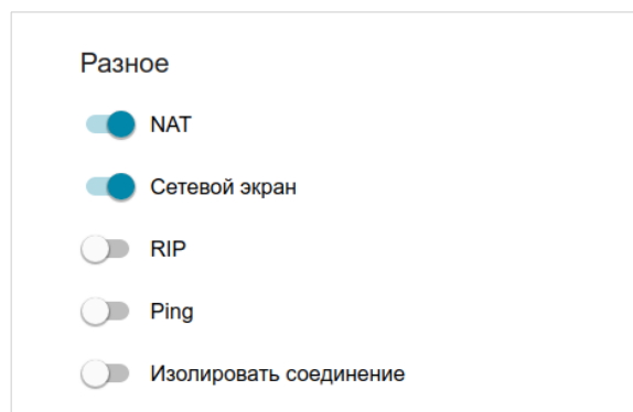
Рисунок 68. Страница добавления соединения типа PPTP . Раздел Разное .
