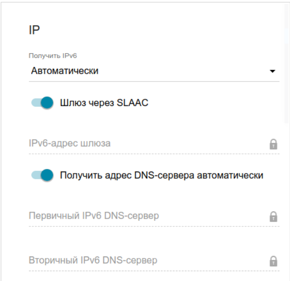
Рисунок 72. Страница добавления соединения типа PPPoE IPv6. Раздел IP.
