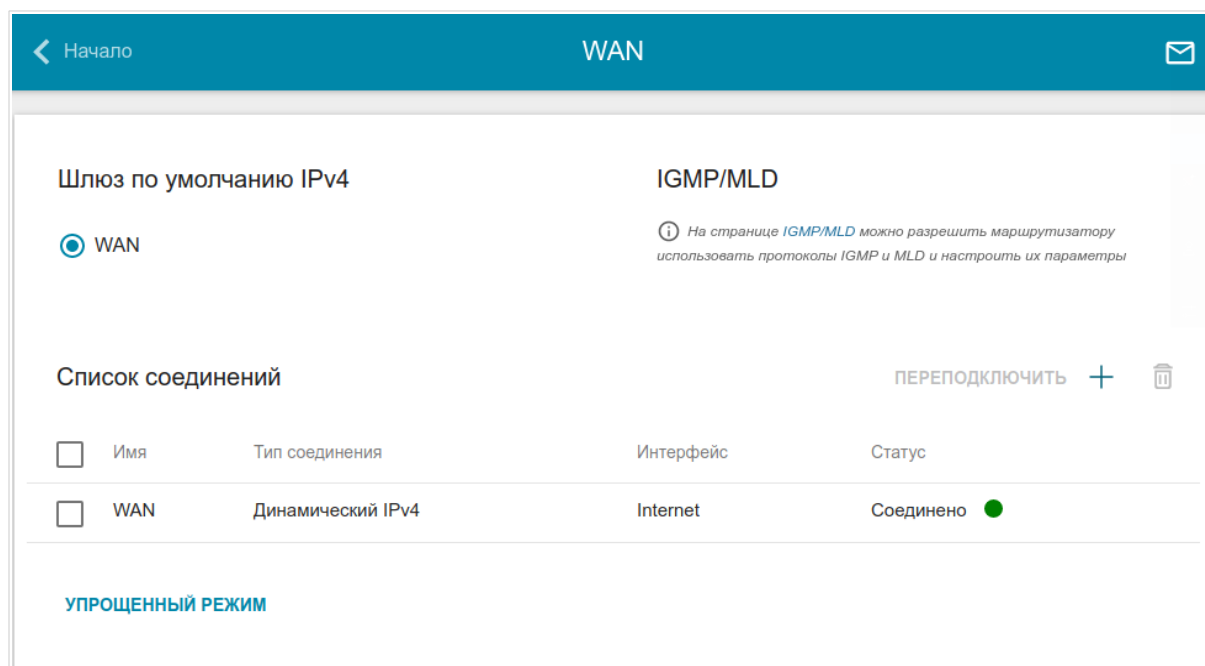
Рисунок 52. Страница Настройка соединений / WAN . Расширенный режим.
