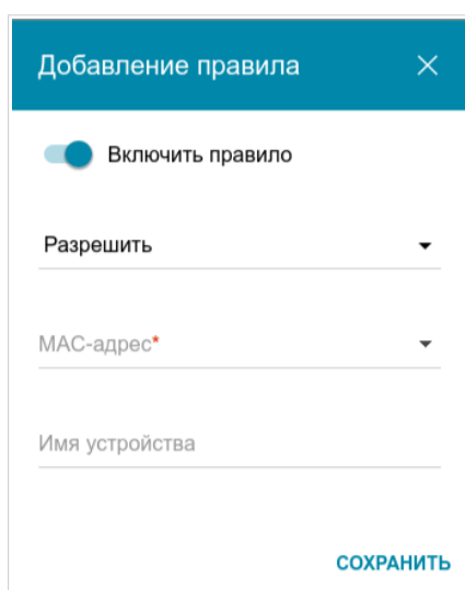
Рисунок 131. Окно добавления правила для MAC-фильтра.
