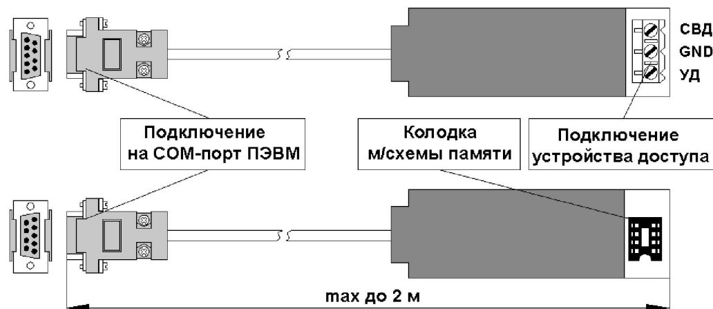
Рисунок 35 – Внешний вид программатора PROG-1 с возможностью подключения к COM-порту ПЭВМ
