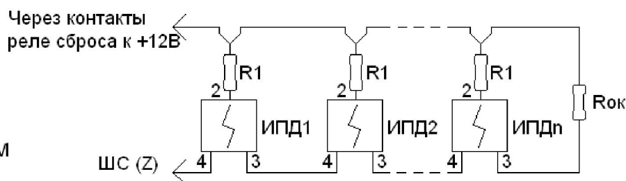
Рисунок 6 - Схема подключения дымовых 2-х проводных извещателей ИПД12 моделей 5М, 44, 54Т, 3СУ, 41М в пожарный ШС с контролем 5-ти состояний
