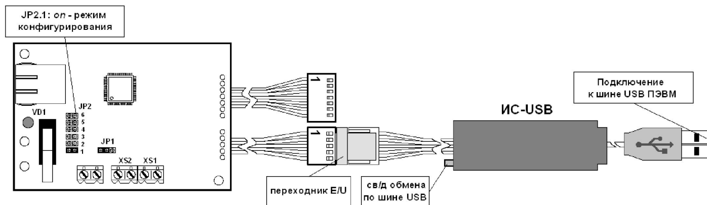
Рисунок 27 – Подключение модулей IC-ETH/485 и IC-USB.
