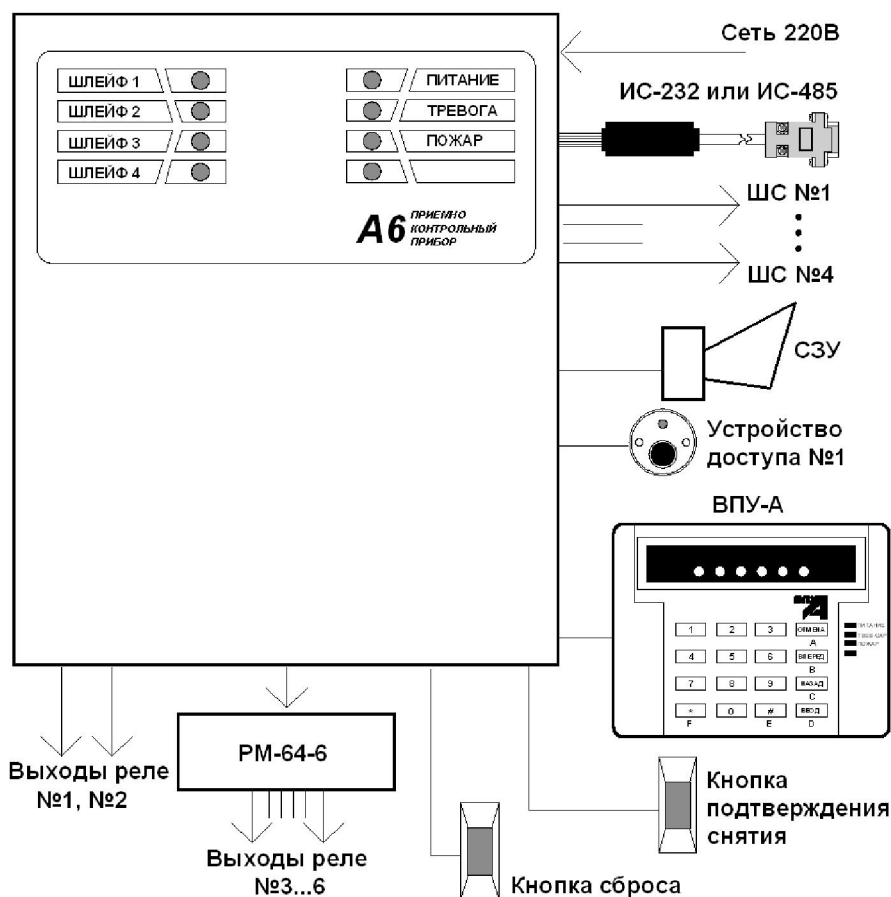
Рисунок 3 – Внешний вид прибора «А6» (исполнение А6-04)
