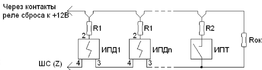
Рисунок 8 - Схема подключения дымовых 2-х проводных извещателей ИПД12 моделей 5М, 44, 54Т, 3СУ, 41М и тепловых извещателей с нормально разомкнутыми контактами в один пожарный ШС с контролем 5-ти состояний
