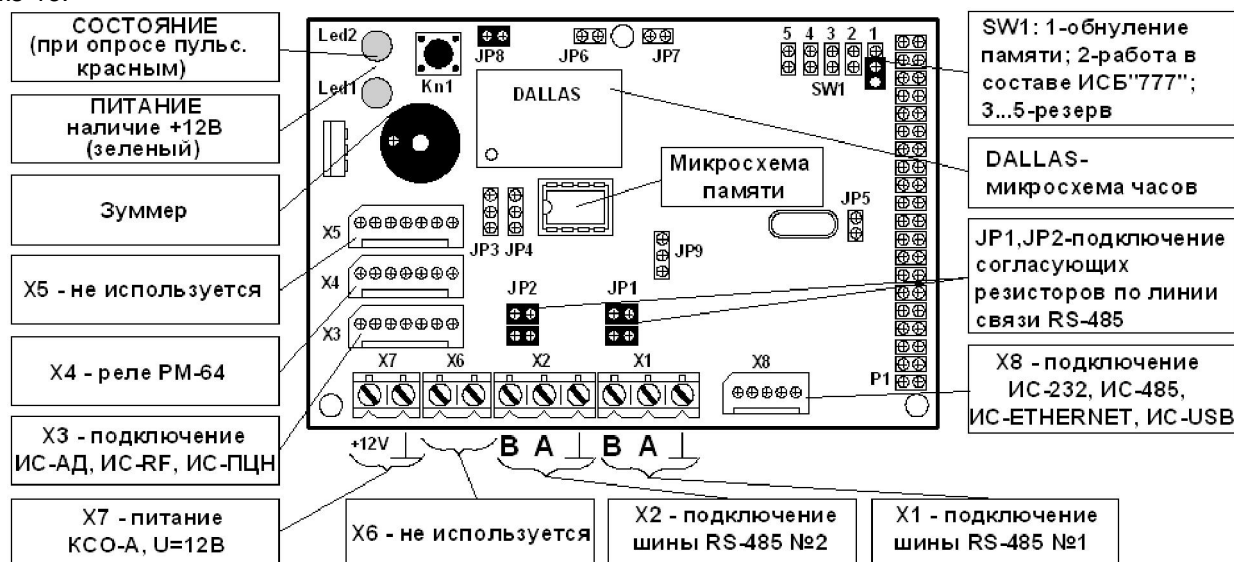
Рисунок 15 – Внешний вид модуля процессорного КСО-А
