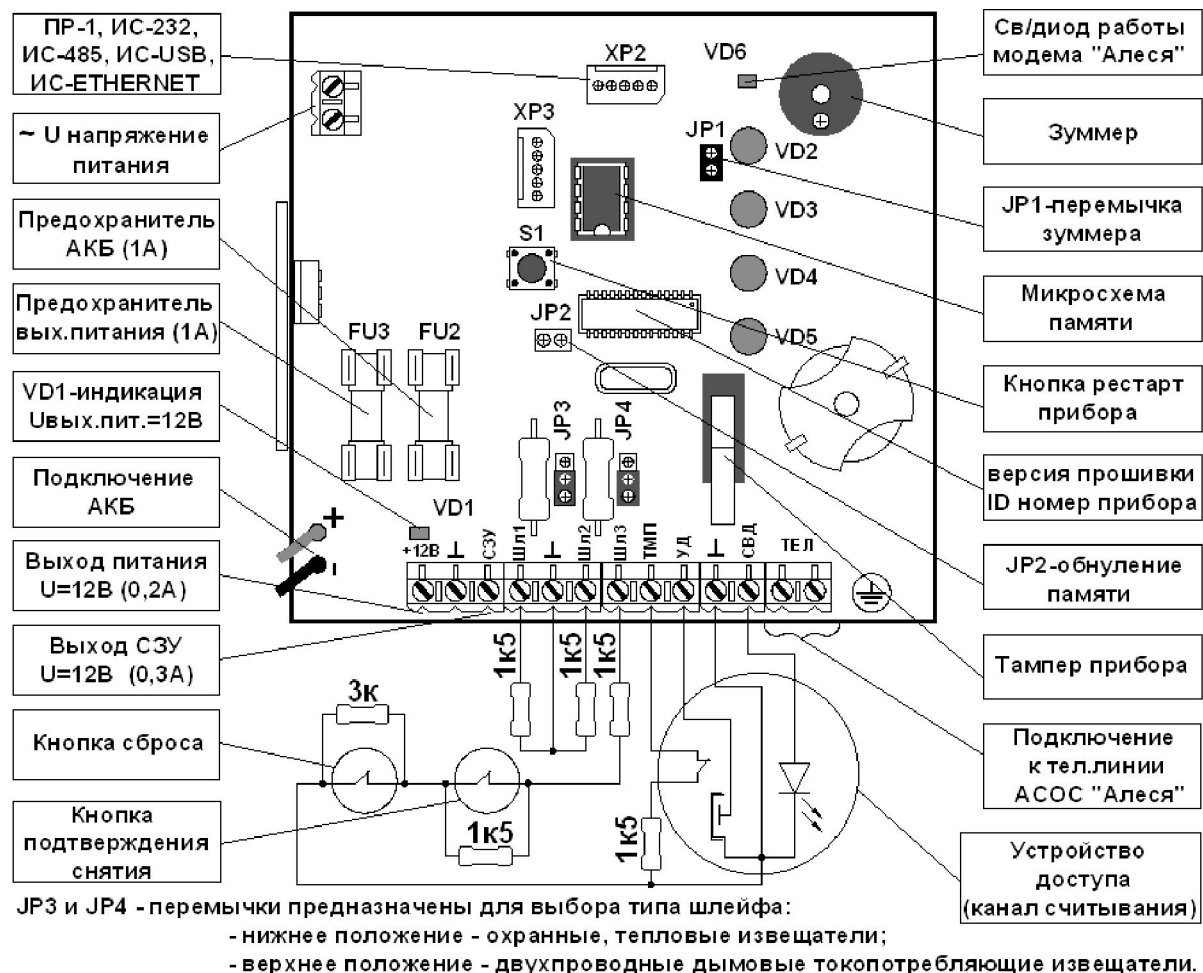
Рисунок 2 – Внешний вид платы управления прибора «А6» исполнения А6-02А
