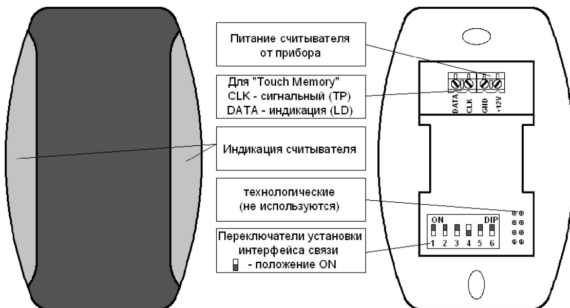
Рисунок 6 – Внешний вид выносной контрольной панели ВКП
