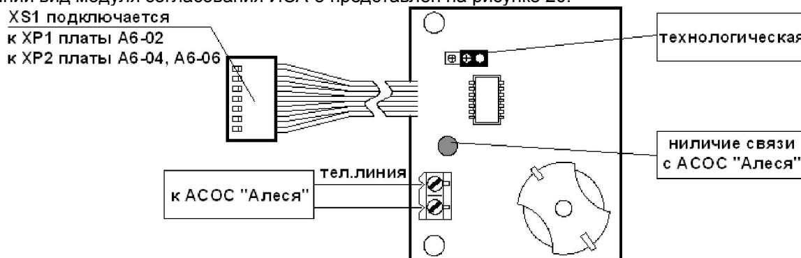
Рисунок 20 – Внешний вид модуля согласования ИСА-8
