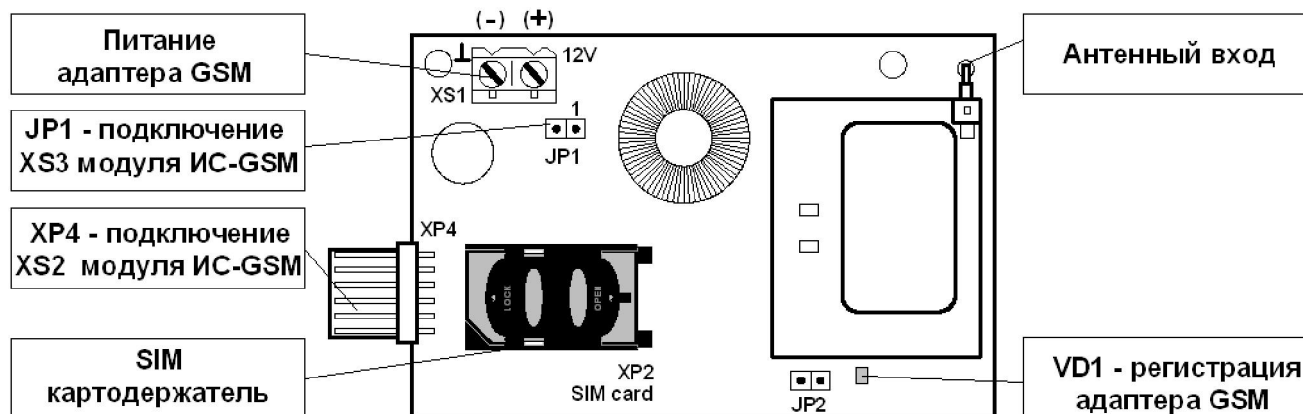
Рисунок 32 - Внешний вид адаптера GSM
