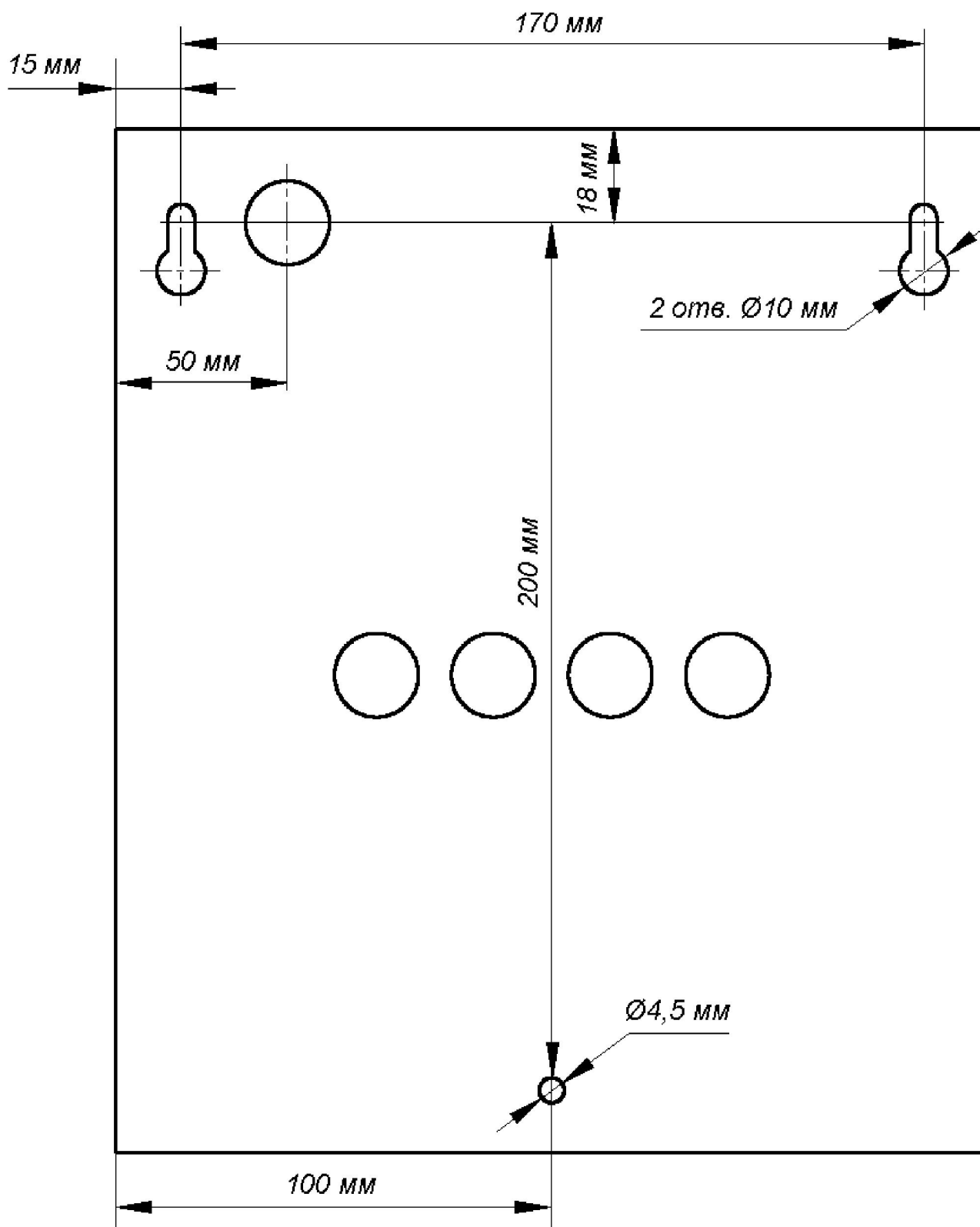
Рисунок 1 – Установочный эскиз прибора «А6»
