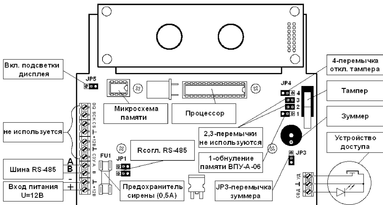
Рисунок 11 - Внешний вид клавиатуры ВПУ-А-06 со снятой задней крышкой
