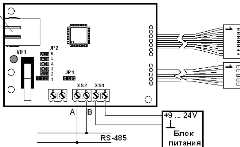
Рисунок 26 – Подключение модуля IC-ETH/485 к RS-485.
