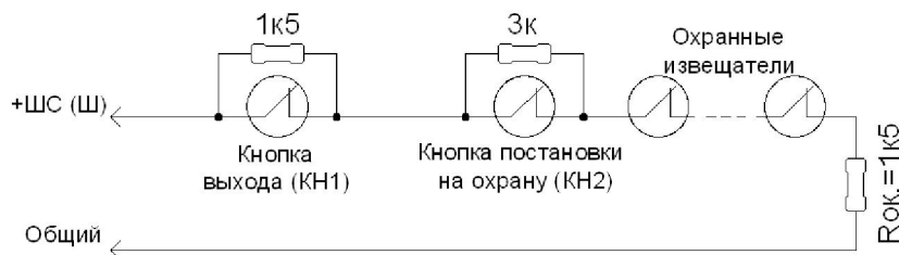
Рисунок 337 – Подключение в шлейф «Кнопки постановки на охрану» и «Кнопки выхода»
