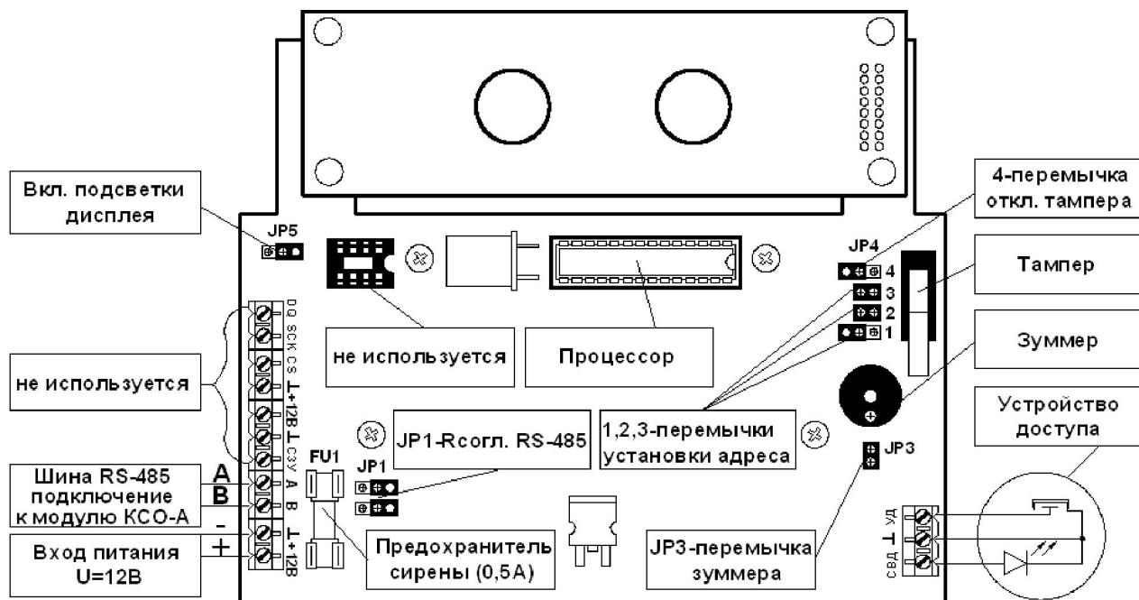
Рисунок 12 - Внешний вид клавиатуры ВПУ-А-16 со снятой задней крышкой
