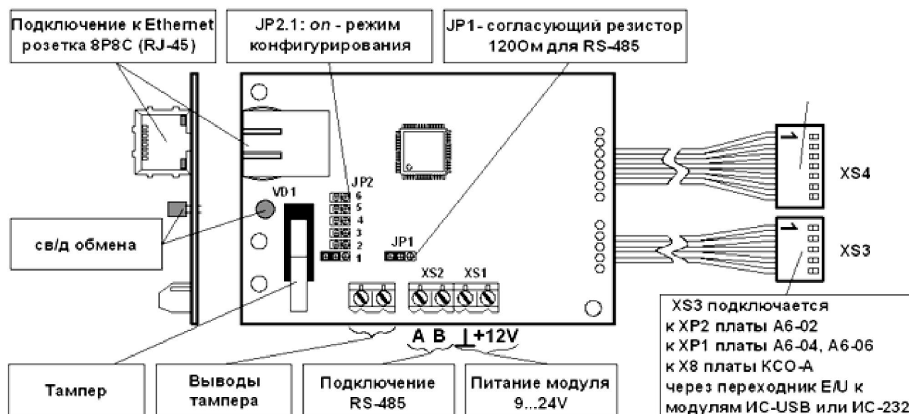
Рисунок 25 – Внешний вид модуля ИС-ЕТН/485.
