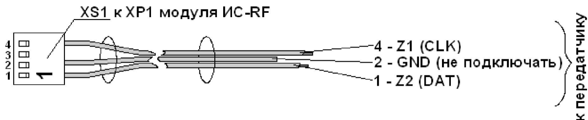
Рисунок 2 – Внешний вид шлейфа-адаптера при работе прибора «А6» в составе РСПИ «ИРБИС» («Cortex»)
