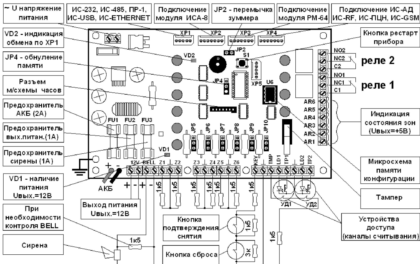
Рисунок 3 – Внешний вид платы управления прибора «А6» исполнения А6-04
