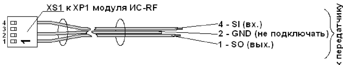
Рисунок 3 – Внешний вид шлейфа-адаптера при работе прибора «А6» в составе РСПИ «LARS» (KP Electronic Systems)
