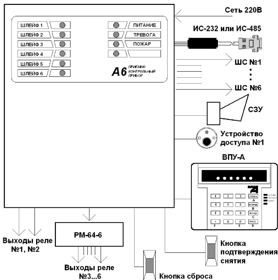
Рисунок 4 – Внешний вид прибора «А6» (исполнение А6-06)
