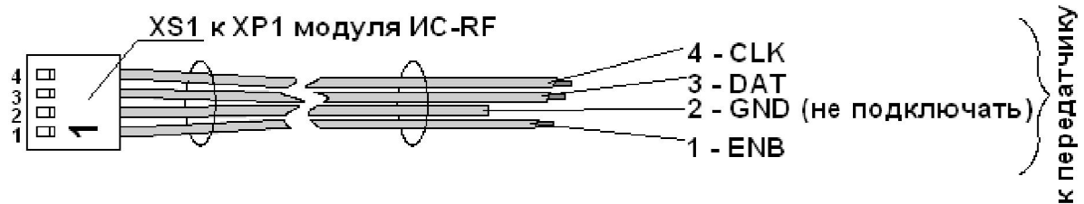
Рисунок 4 – Внешний вид шлейфа-адаптера при работе прибора «А6» в составе РСПИ «Андромеда» («PIMA»)
