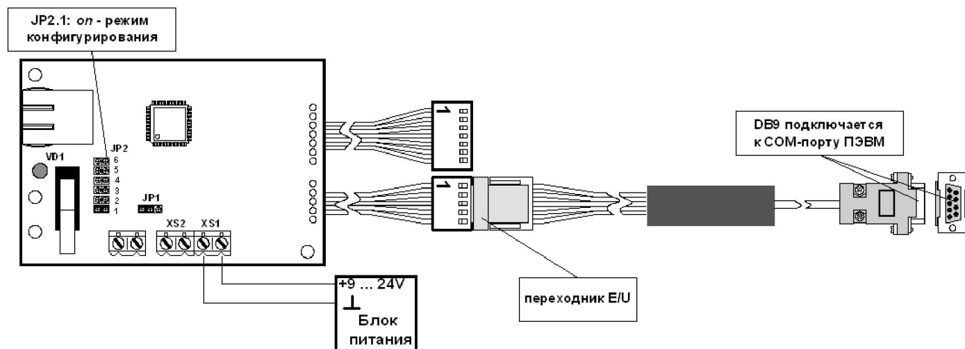
Рисунок 28 – Подключение модулей ИС-ЕТН/485 и ИС-232
