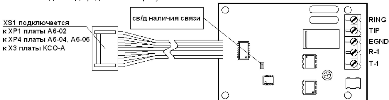
Рисунок 24 – Внешний вид модуля согласования ИС-АД
