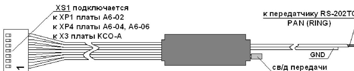
Рисунок 23 – Внешний вид модуля согласования ИС-ПЦН
