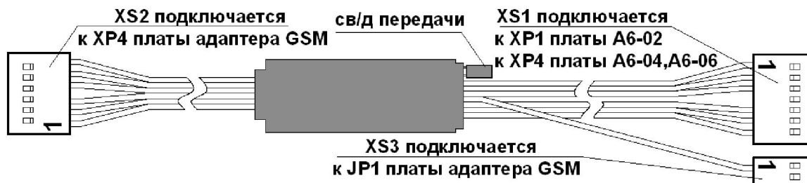
Рисунок 31 - Внешний вид модуля согласования ИС-GSM
