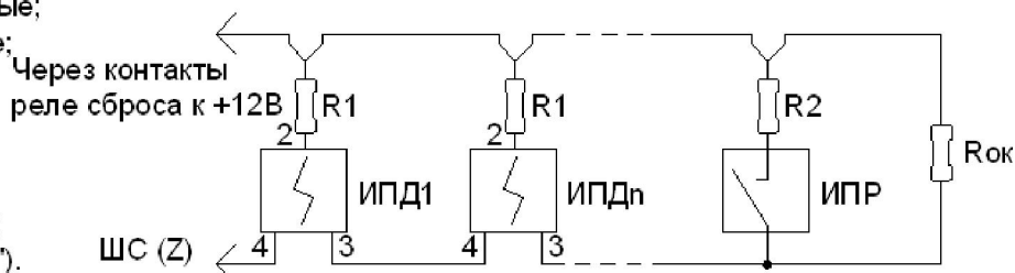
Рисунок 9 - Схема подключения дымовых 2-х проводных извещателей ИПД12 моделей 5М, 44, 54Т, 3СУ, 41М и ручных извещателей с нормально разомкнутыми контактами в один пожарный ШС с контролем 5-ти состояний
