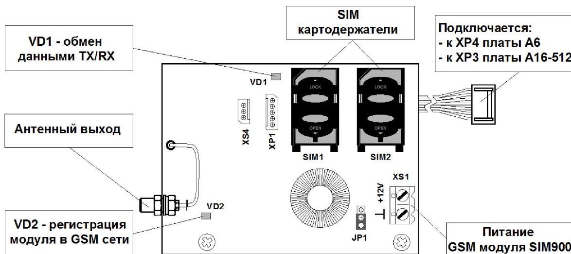
Рисунок 30 – Адаптер GSM (на 2 SIM-карты)
