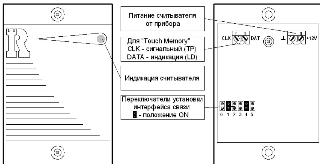
Рисунок 5 – Внешний вид выносной контрольной панели ВКП
