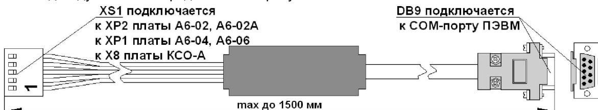
Рисунок 18 – Внешний вид модуля согласования IC-232
