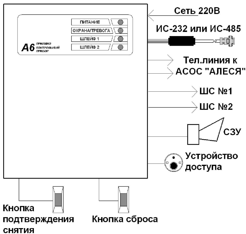
Рисунок 2 – Внешний вид прибора «А6» (исполнение А6-02А)
