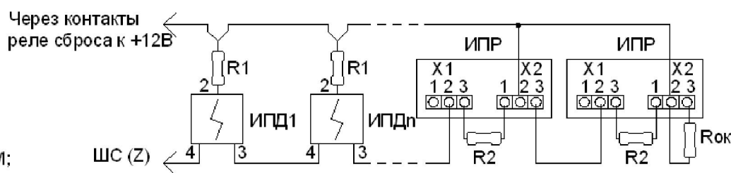
Рисунок 10 - Схема подключения ручных извещателей ИПР-3СУ и ИП5-2Р в пожарный ШС совместно с дымовыми 2-х проводными извещателями ИПД12 моделей 5М, 44, 54Т, 3СУ, 41М.
