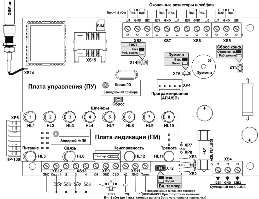
Рисунок 1 - Плата управления
