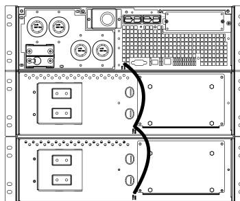
Соединения проводников заземления для подавления выбросов напряжения
