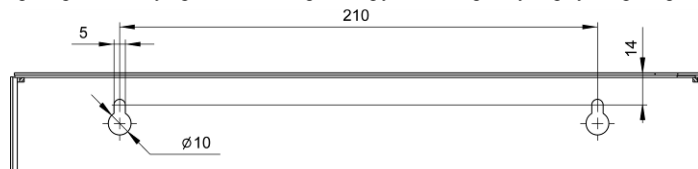
Рисунок 6 – Элементы крепления корпуса прибора ПКП-128
